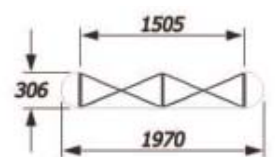
3x2 - Droit 2 lès centrales + 2 retour
