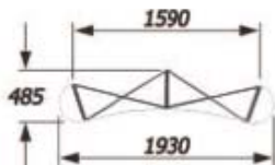
3x2 - Courbe 2 lès centrales + 2 retour
