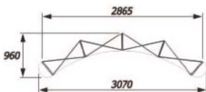
3x4 - Courbe 4 lès centrales + 2 retour
