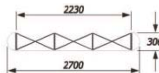
3x3 - Droit 3 lès centrales + 2 retour
