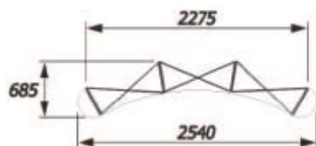
3x4 - Courbe 4 lès centrales + 2 retour
